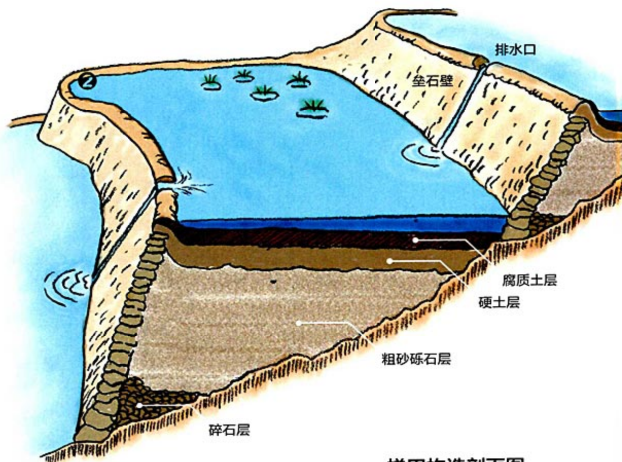
梯田构造剖面图
