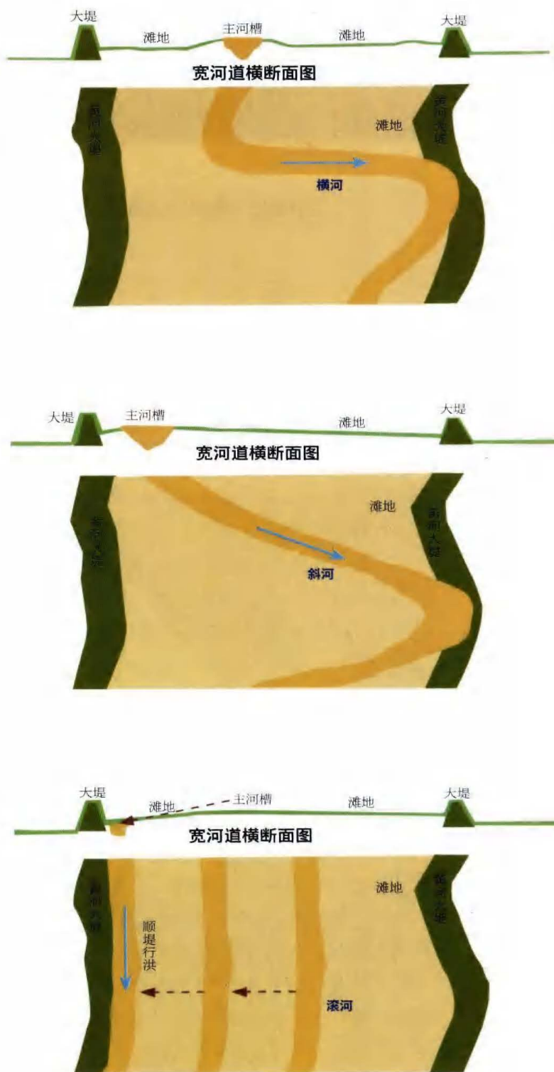
黄河下游河道“横河”“斜河”“滚河”示意图
