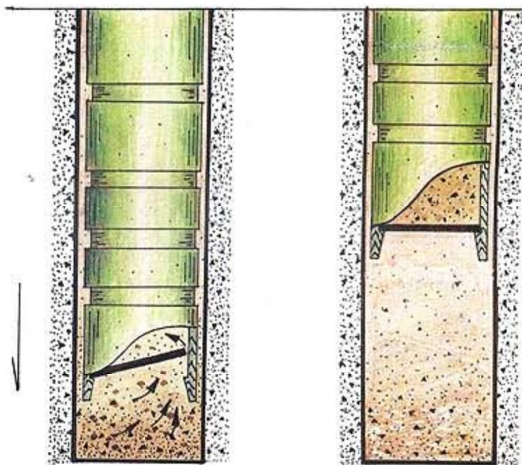
卓筒井掘井原理图
