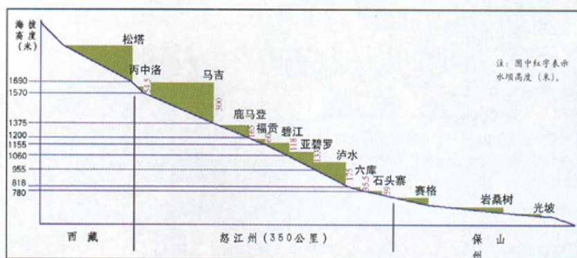
怒江州水电梯级开发示意图
