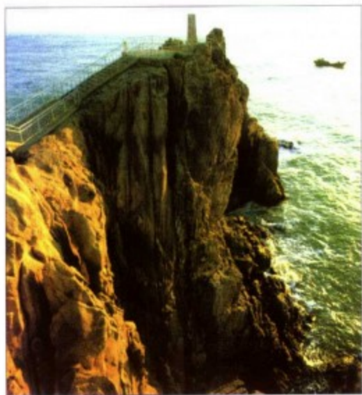
成山头山石巍峨峻峭，如巨龙翘首大海。
