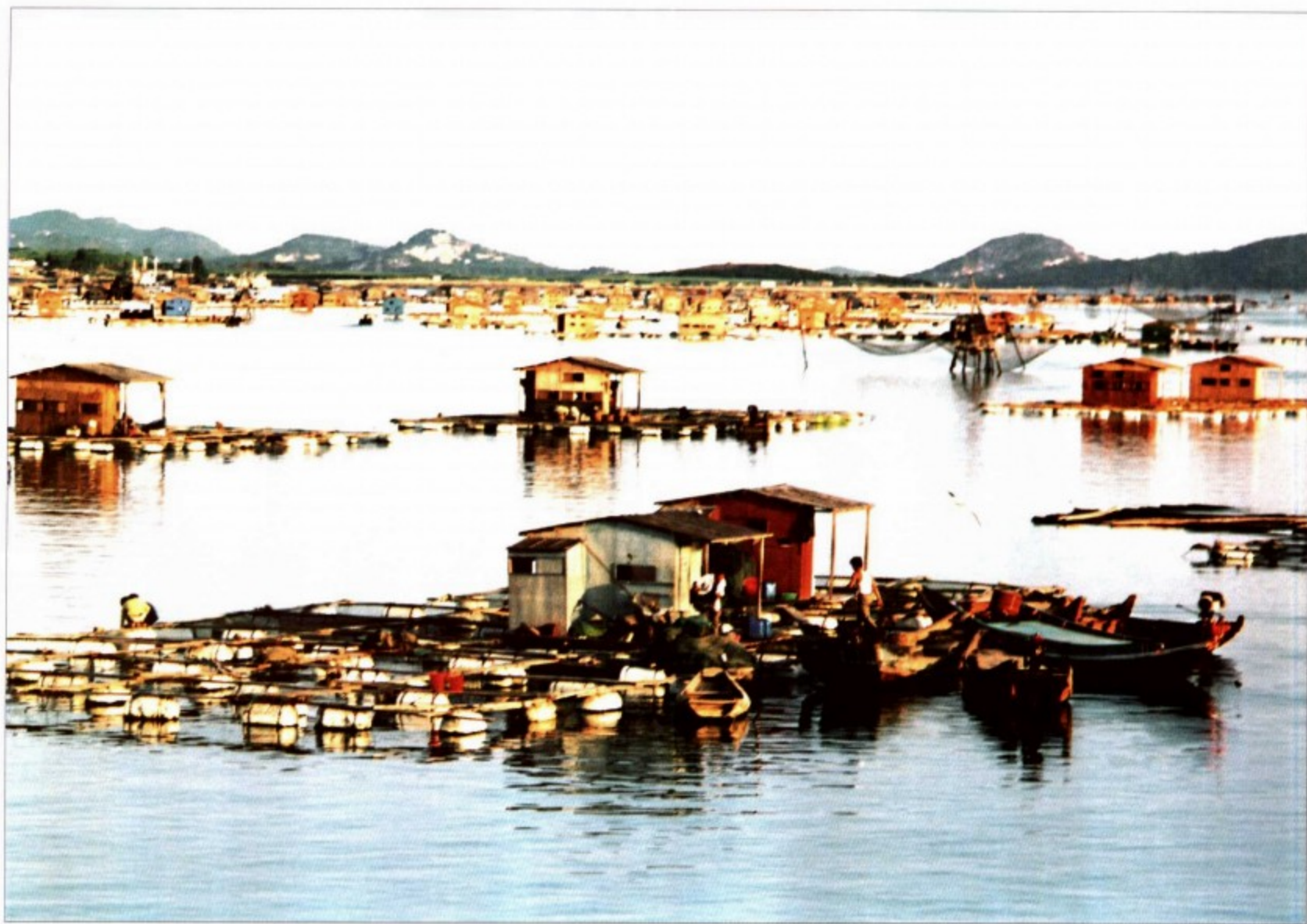
东山岛八尺门“海上牧场”，人工养殖了各种名贵的海产品，也是东山岛的旅游一景。
