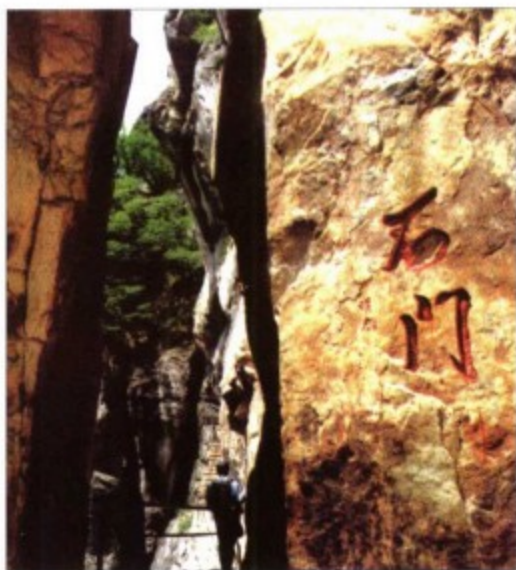
攀登嵩山的必经之路——石门
