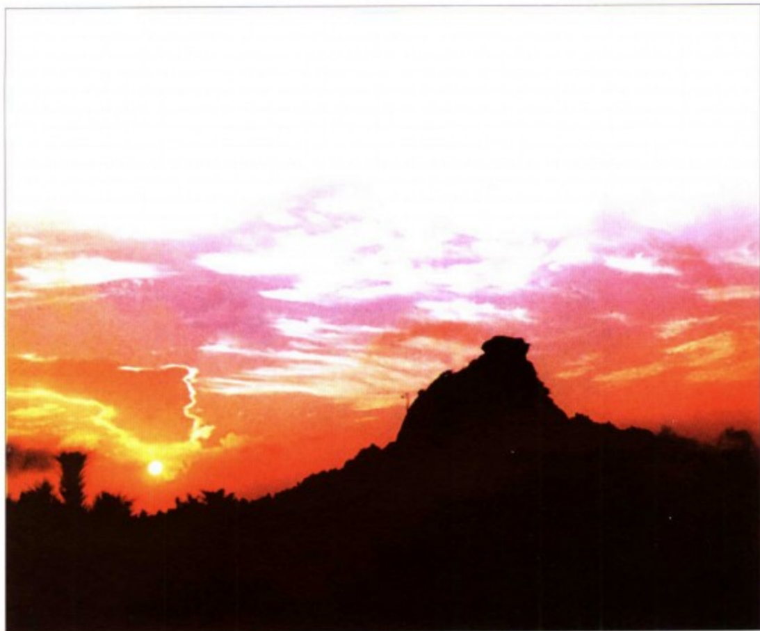
晨曦中的鸡公山就宛如雄鸡报晓。
