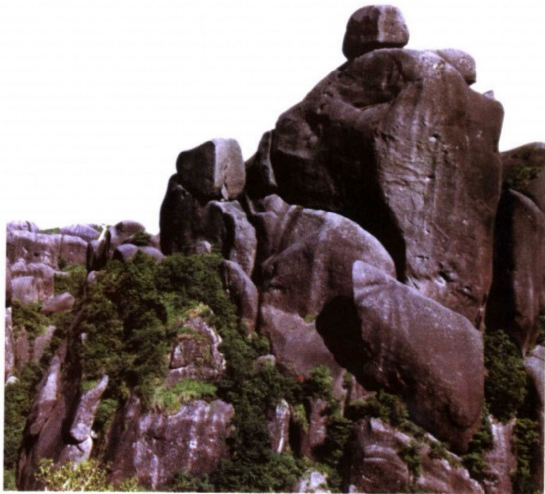
太姥山无俗石，每一块石头都栩栩如生。
