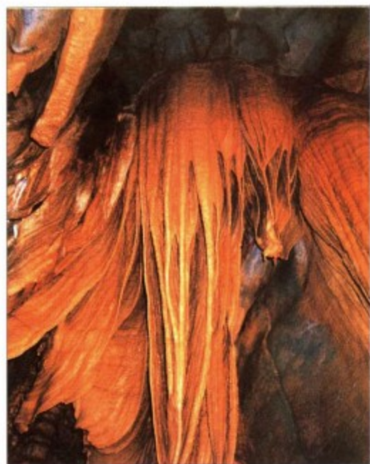
江南溶洞群中的著名溶洞——鱼龙洞
