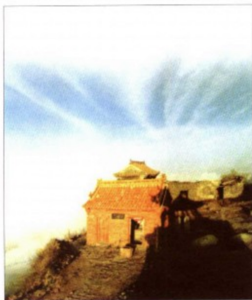
王屋山的天坛峰上有轩辕黄帝祭天处等人文胜迹。
