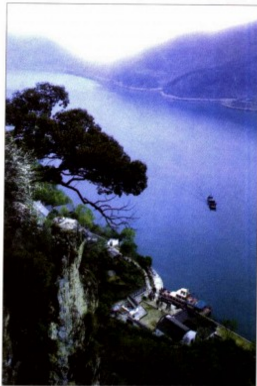
风光旖旎的富春江
