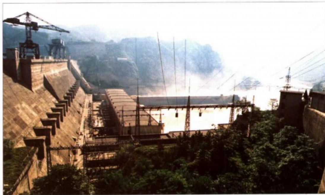
1957年在三门峡建起高106米，长875米的拦河大坝，使高峡变成了平湖。
